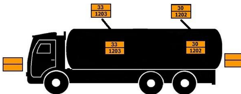
Imagen 3.8.6.5: Señalización de vehículos
