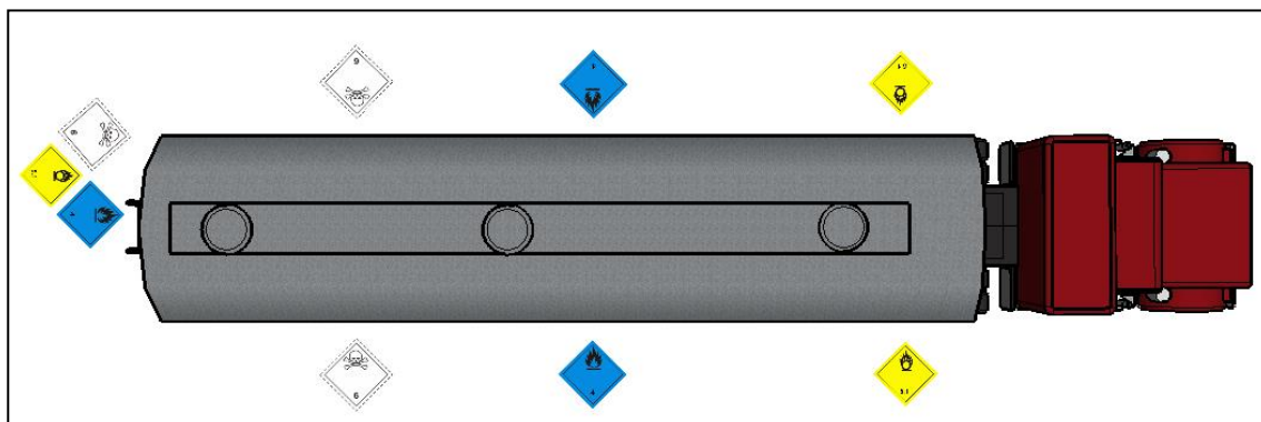
Imagen 3.8.1.5: Etiquetado compartimentos múltiples
