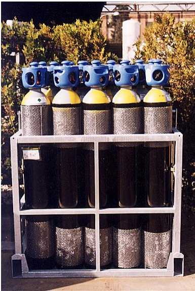
Imagen 3.6.1.1.61: Jaulas para recipientes
