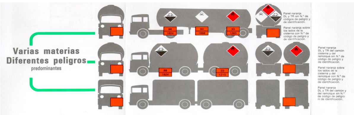
Imagen 3.8.6.2: Señalización de vehículos
