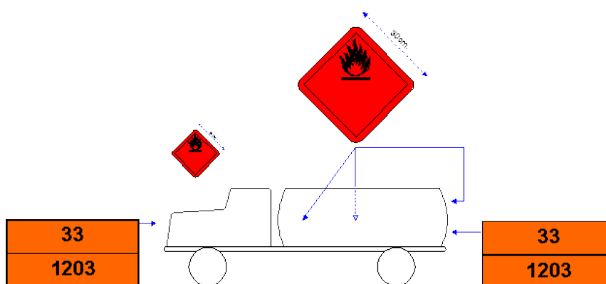
Imagen 3.8.6.6: Señalización de vehículos
