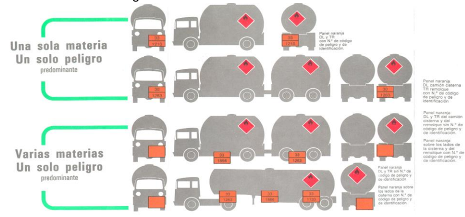
Imagen 3.8.6.1: Señalización de vehículos
