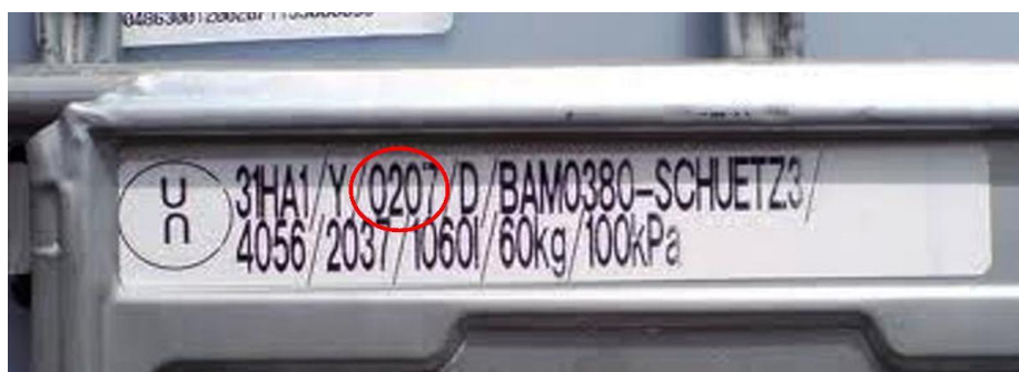
Imagen 3.6.1.2.14: Marcado de GRG
