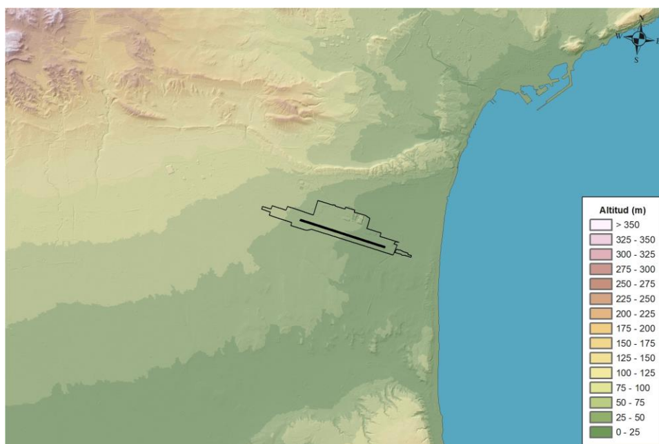
Ilustración 4.1 Modelo digital del terreno. Aeropuerto de Alicante-Elche Miguel Hernández
