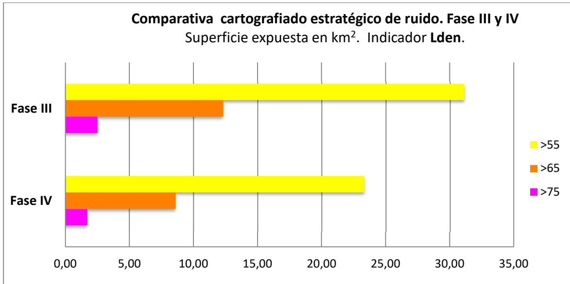
Ilustración 6.5 Comparativa de los valores totales de afección del cartografiado estratégico de ruido. Fase III y IV. Superficie (Km 2 ). Indicador L den
