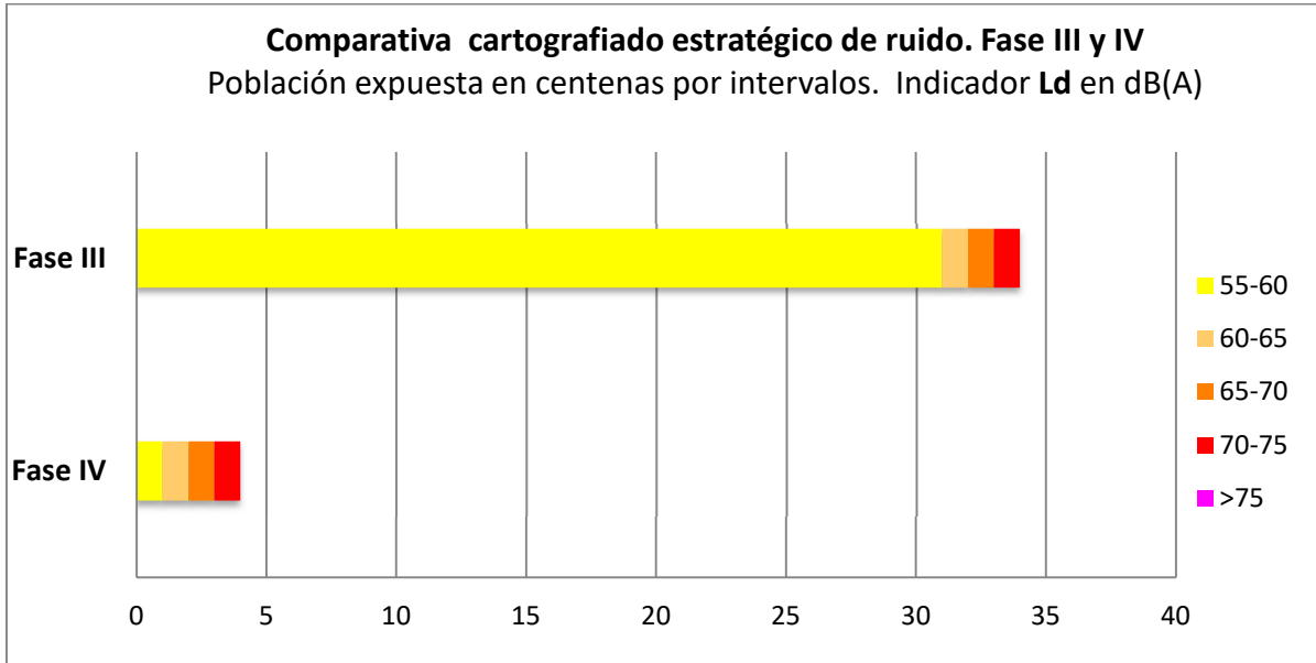
Ilustración 6.3 Comparativa cartografiado estratégico de ruido. Fase III y IV. Población expuesta en centenas. Indicador L d
