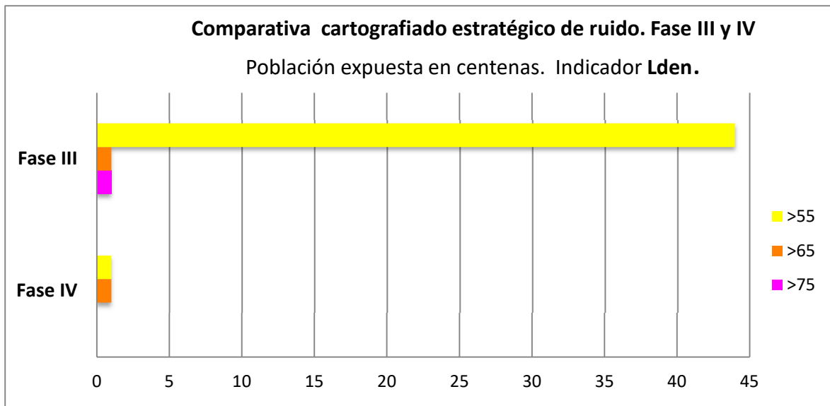
Ilustración 6.6 Comparativa de los valores totales de afección del cartografiado estratégico de ruido. Fase III y IV. Población expuesta en centenas. Indicador L den
