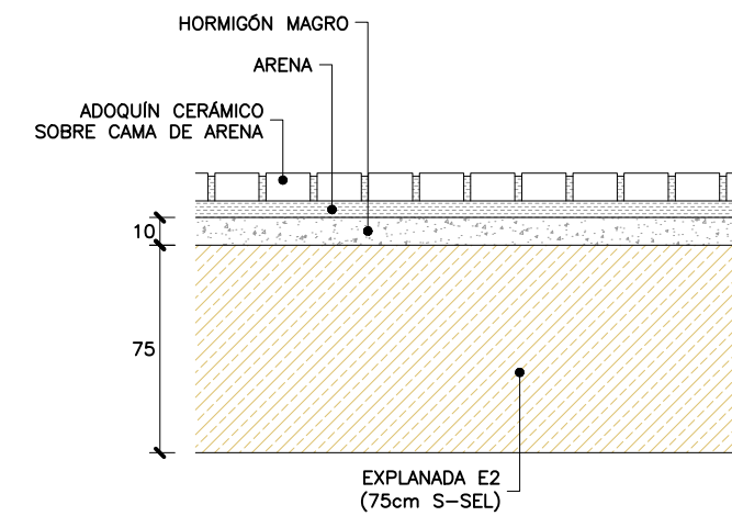
ACERA PEATONAL ESCALA 1/15 Cotas en cm
