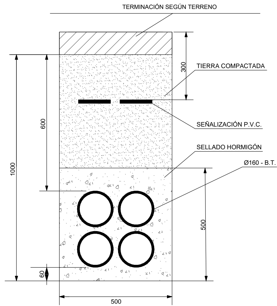
ZANJA 4 TUBOS B.T.
