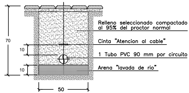
ZANJA EN ACERA
