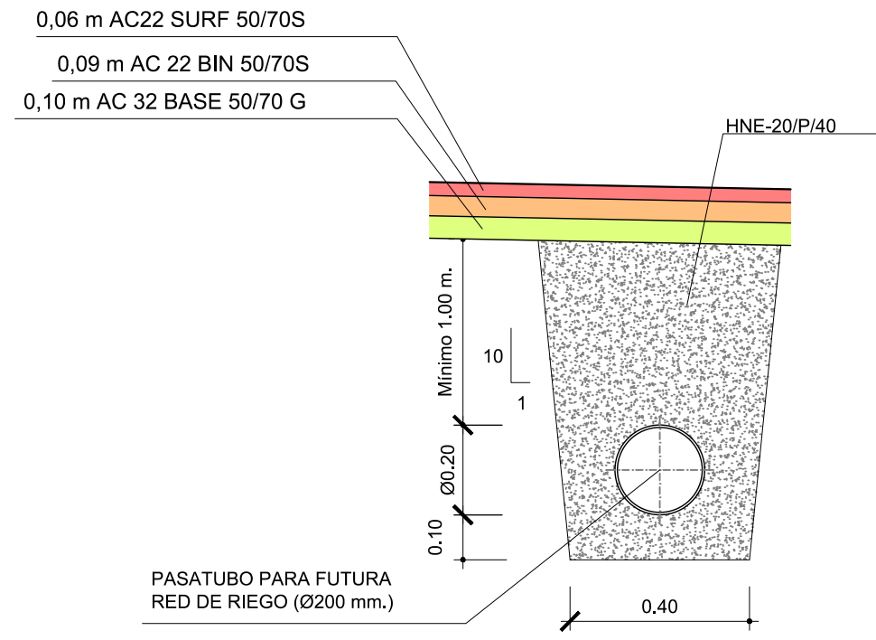
SECCIÓN TIPO DE ZANJA
