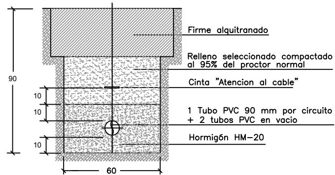
ZANJA EN CRUCE DE CALZADA
