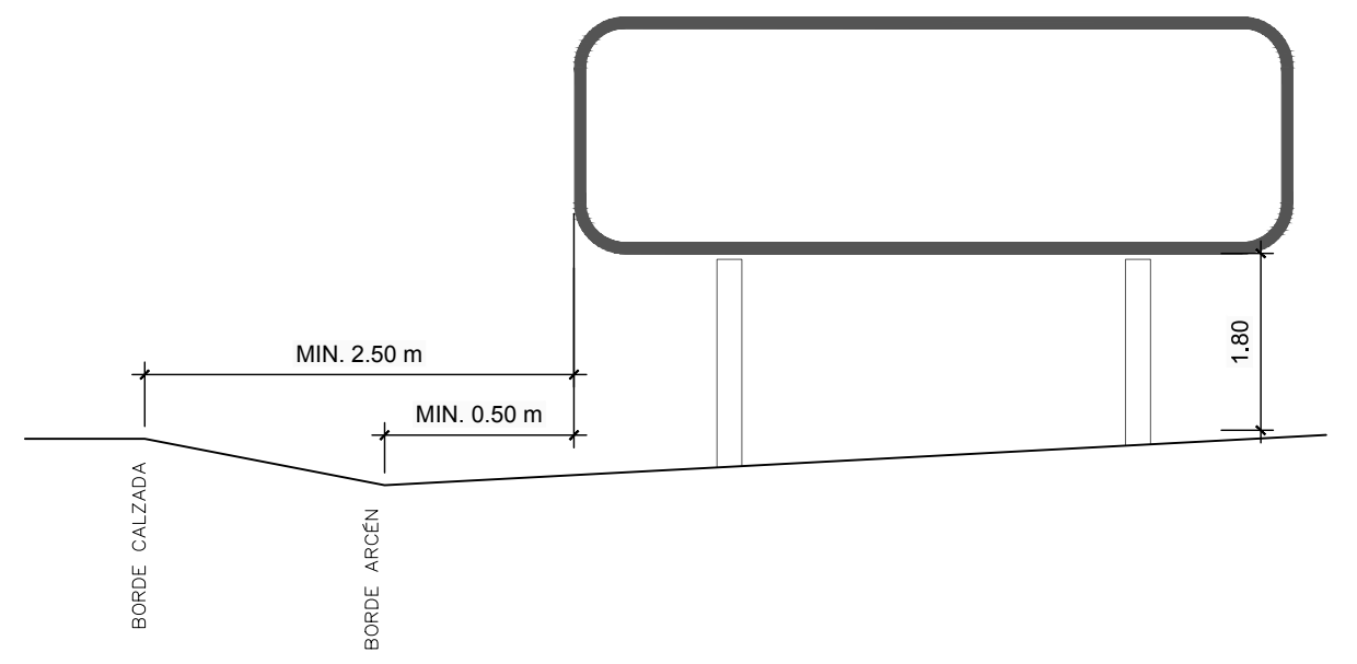
COLOCACIÓN DE SEÑALES VERTICALES
