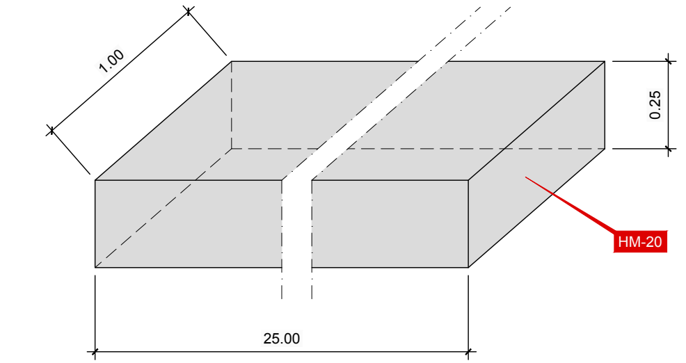
DETALLE DE LOSA DE HORMIGÓN
