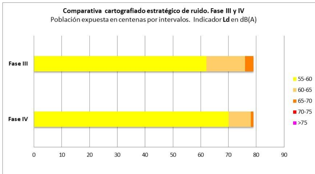
Ilustración 6.3 Comparativa cartografiado estratégico de ruido. Fase III y IV. Población expuesta en centenas. Indicador L_d
