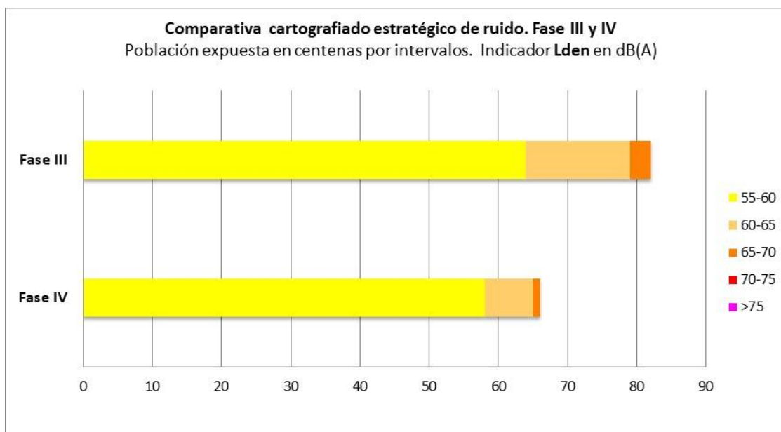
Ilustración 6.1 Comparativa cartografiado estratégico de ruido. Fase III y IV. Población expuesta en centenas. Indicador L_{den}
