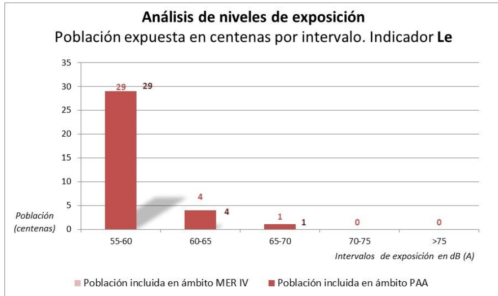
Ilustración 5.4 Valoración de la población que habita en viviendas dentro del ámbito del PAA. Indicador L_e
