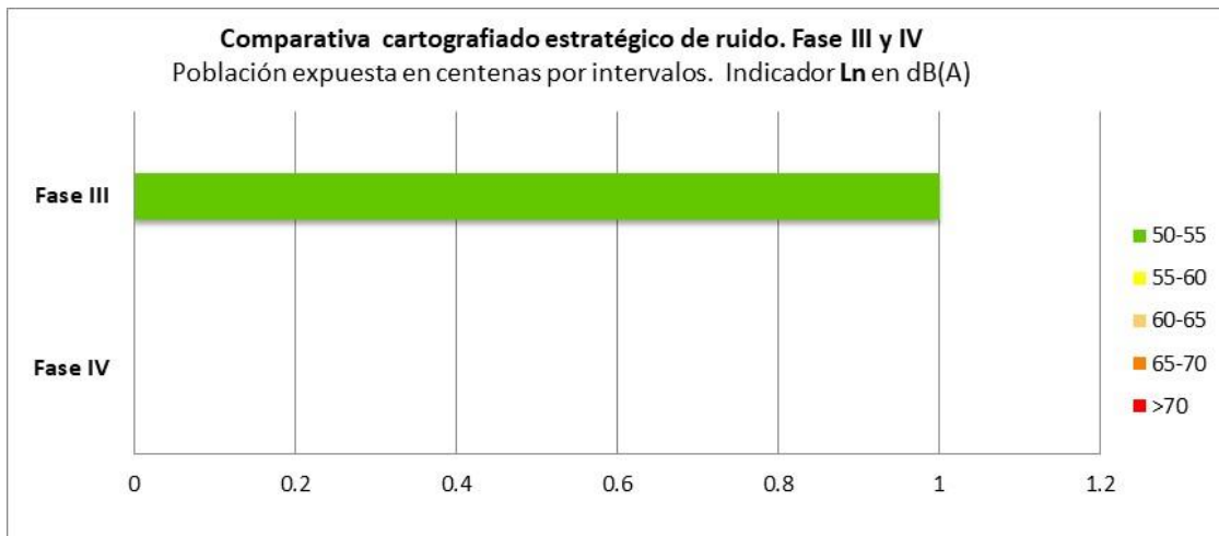
Ilustración 6.2 Comparativa cartografiado estratégico de ruido. Fase III y IV. Población expuesta en centenas. Indicador L_n
