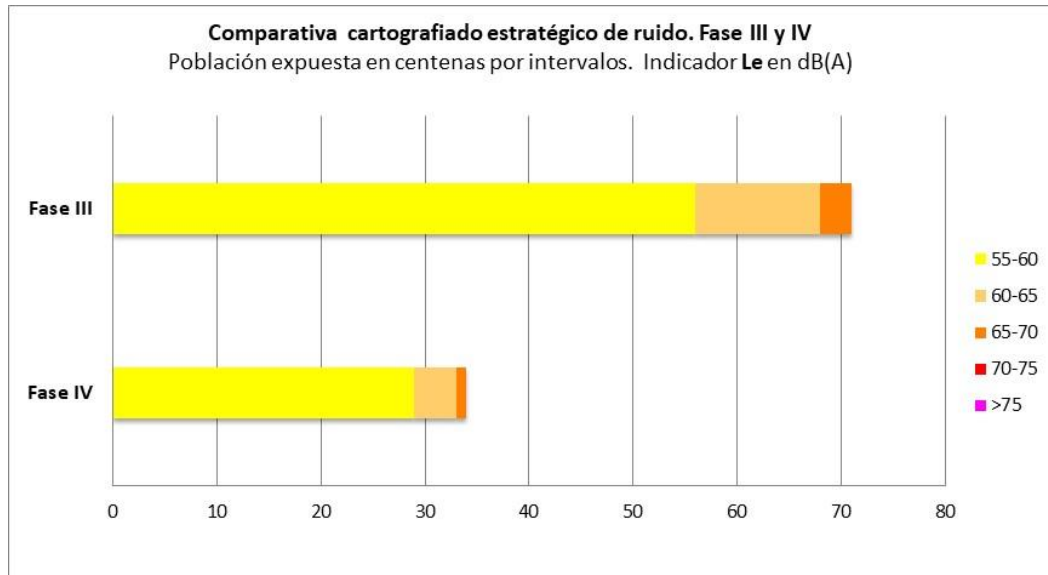
Ilustración 6.4 Comparativa cartografiado estratégico de ruido. Fase III y IV. Población expuesta en centenas. Indicador L_e
