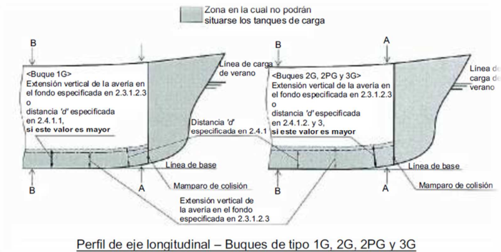
Figura 2.1: Prescripciones relativas a la ubicación de los tanques de carga
