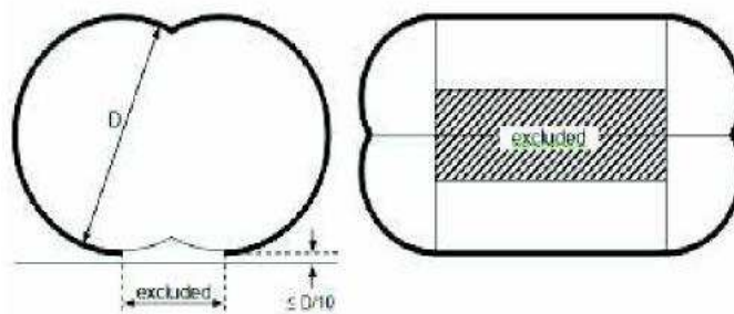
Tanques bilobulares
