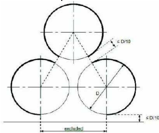
Disposición horizontal de tanques cilíndricos
