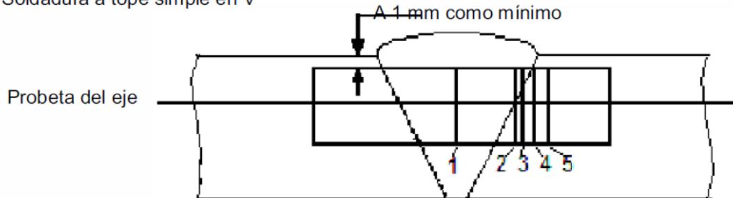
Soldadura a tope simple en V
