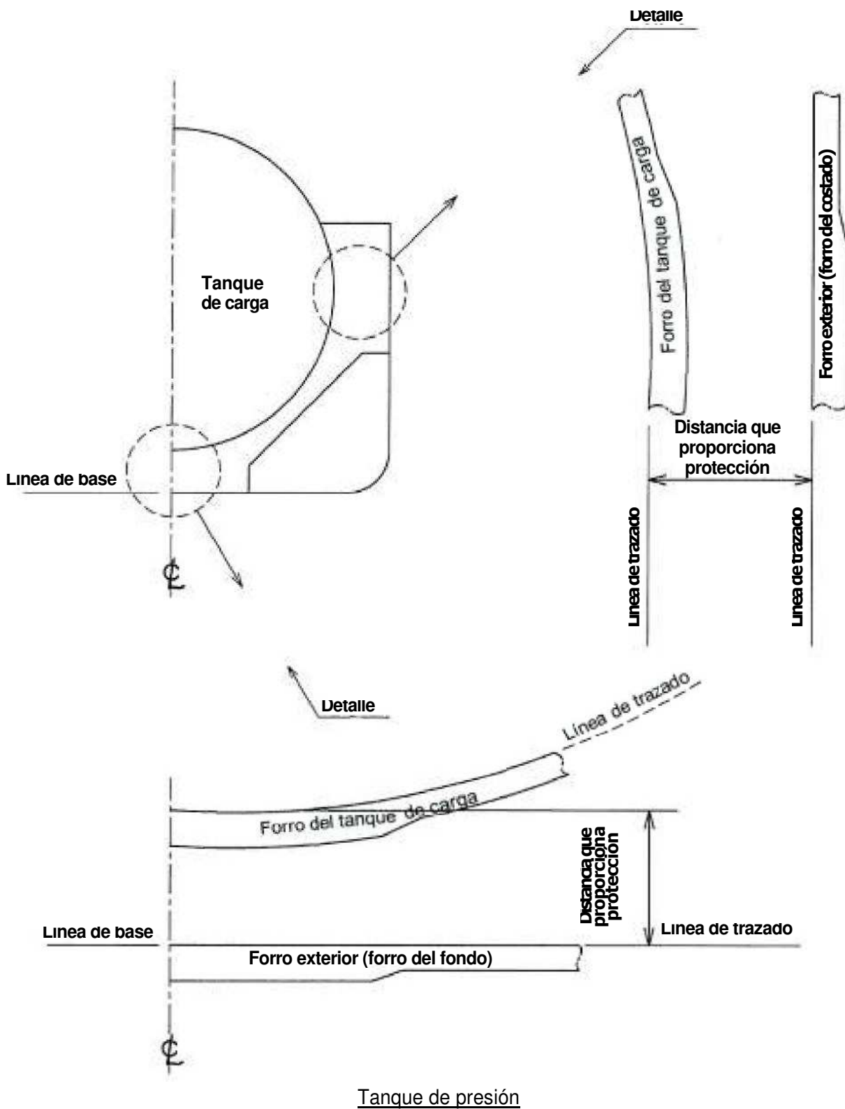
Figura 2.5 e): Distancia que proporciona protección
