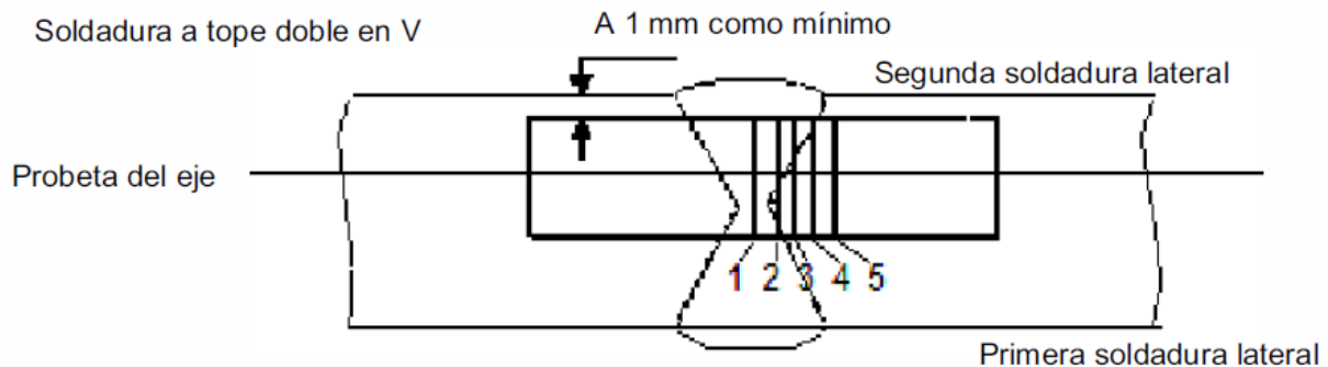
Figura 6.2: Orientación de la probeta de la prueba de soldadura
