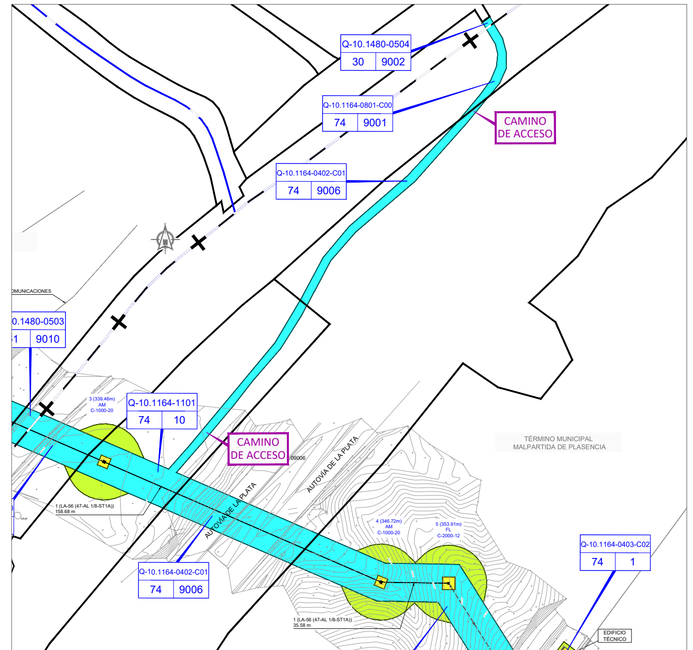
DETALLE 2: CAMINO DE ACCESO AL APOYO Nº3 Escala 1:2000
