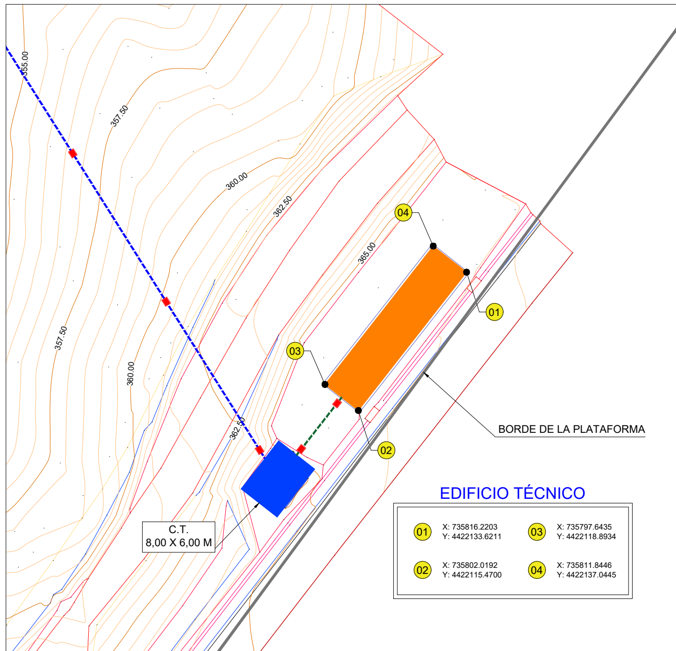
DETALLE 1: EDIFICIO TÉCNICO Escala 1:1500
