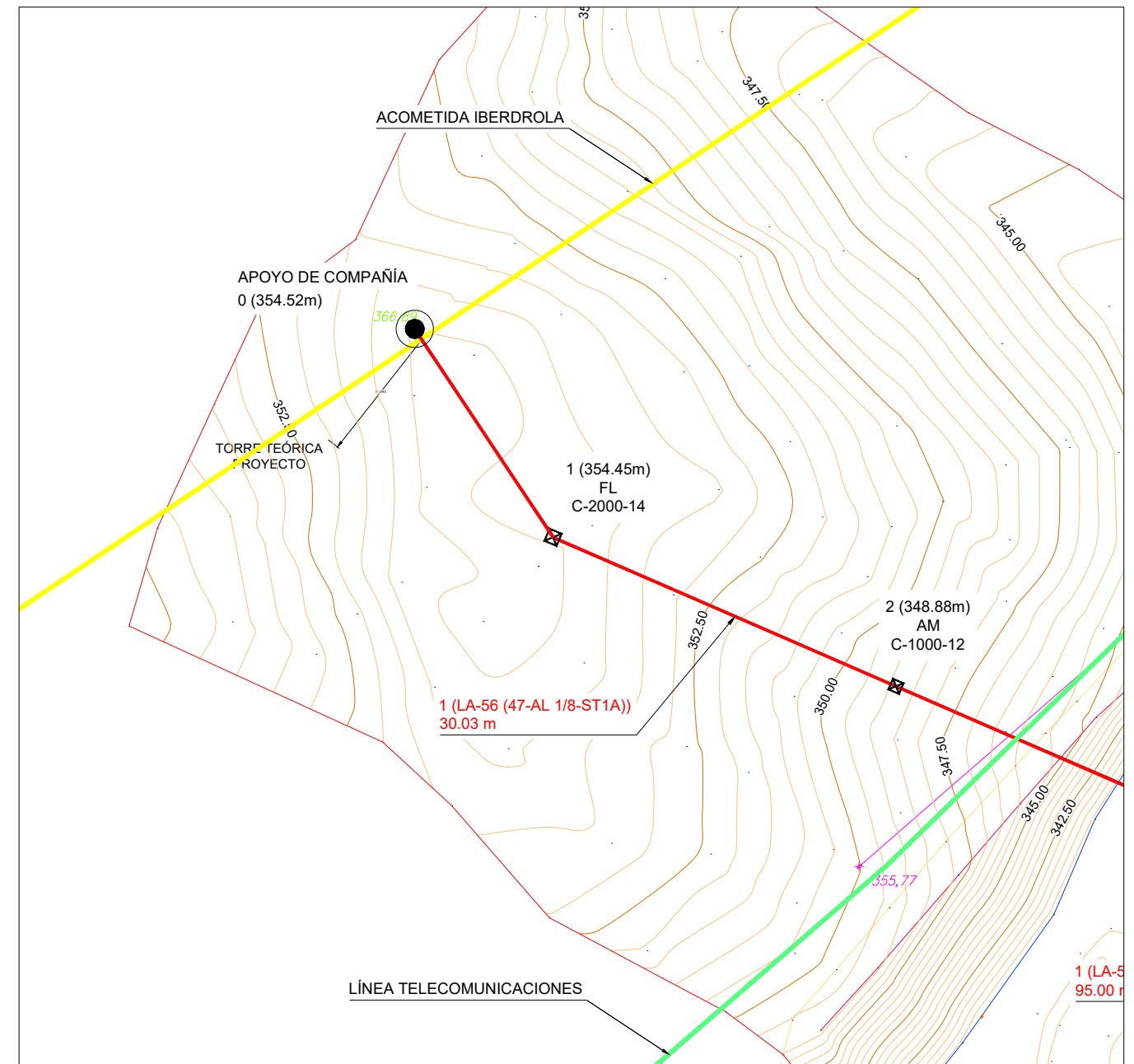
DETALLE 2: PUNTO DE SUMINISTRO Escala 1:1500
