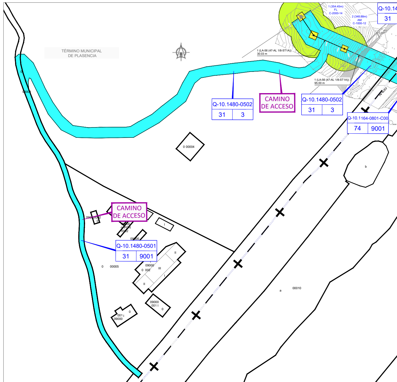
DETALLE 1: CAMINO DE ACCESO AL APOYO DE LA COMPAÑÍA Escala 1:2000
