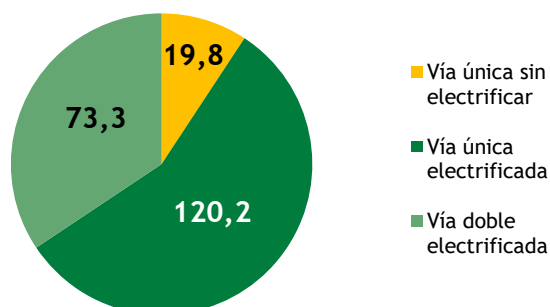
Longitud (km) de la red de ETS según sus características (31-12-2021)
