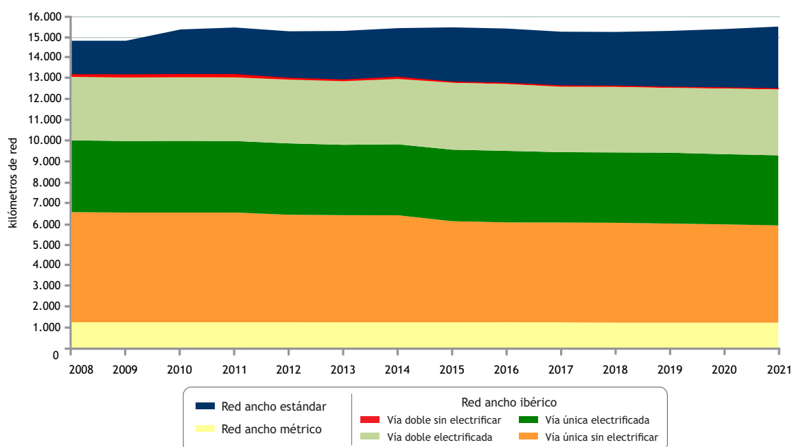
Longitud de las redes según características de la vía en la red gestionada por Adif (2008-2021)
