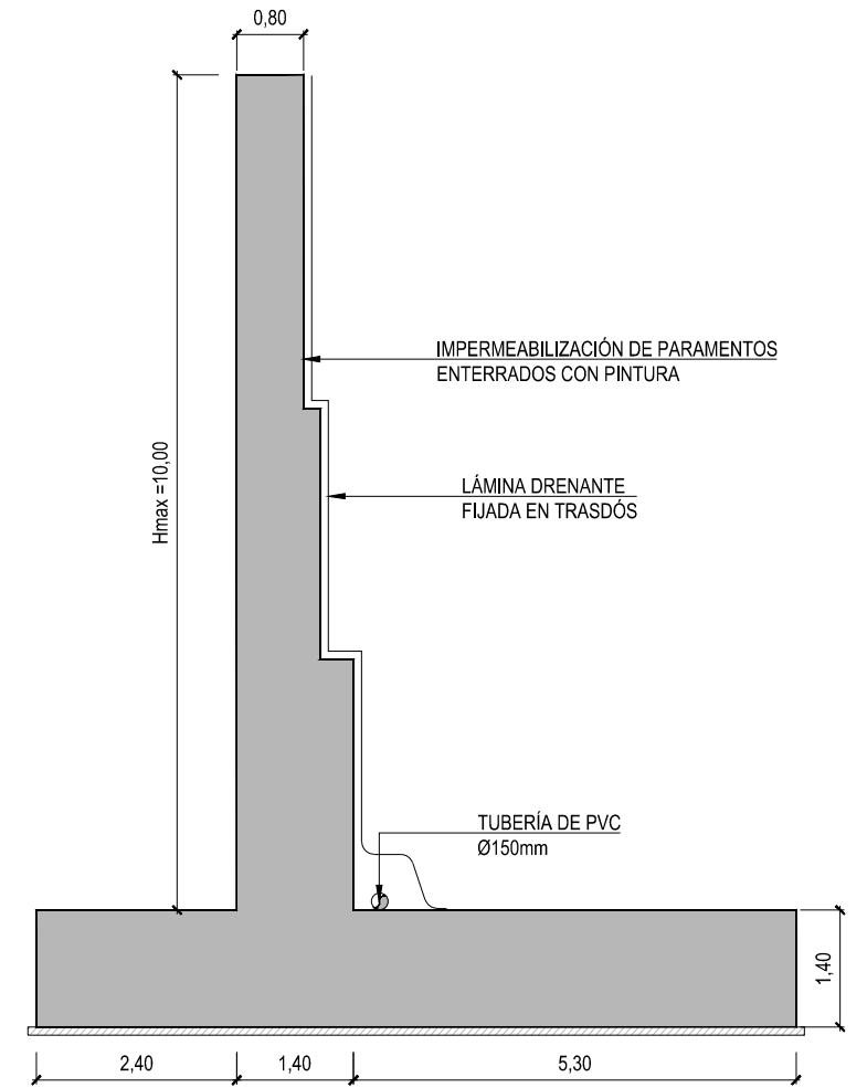
MURO TIPO 3 ESCALA: 1/100
