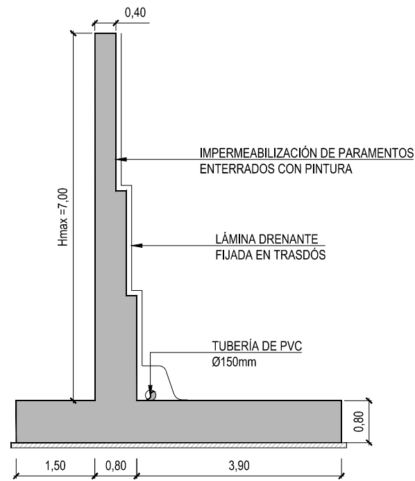
MURO TIPO 2 ESCALA: 1/100
