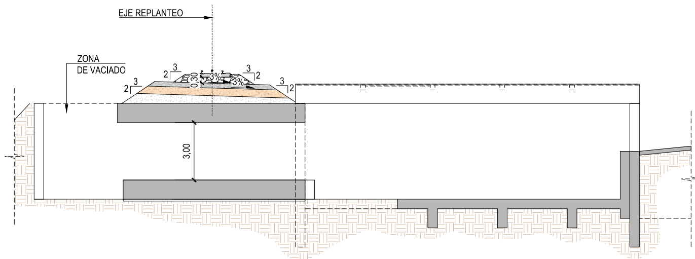
PASO INFERIOR TIPO 1. ALZADO ESCALA: 1/200
