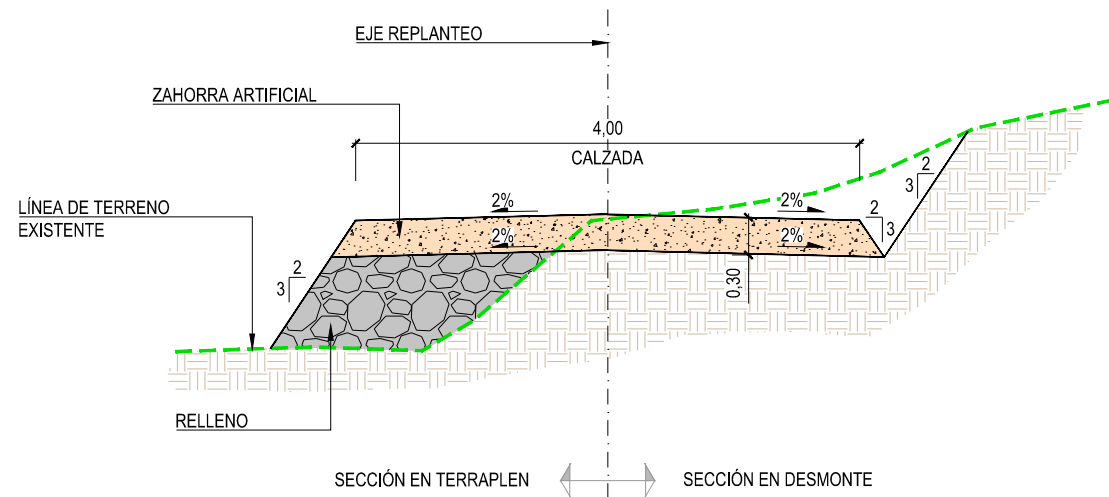
SECCIÓN TIPO: CAMINO (ANCHO = 4m) ESCALA: 1/60
