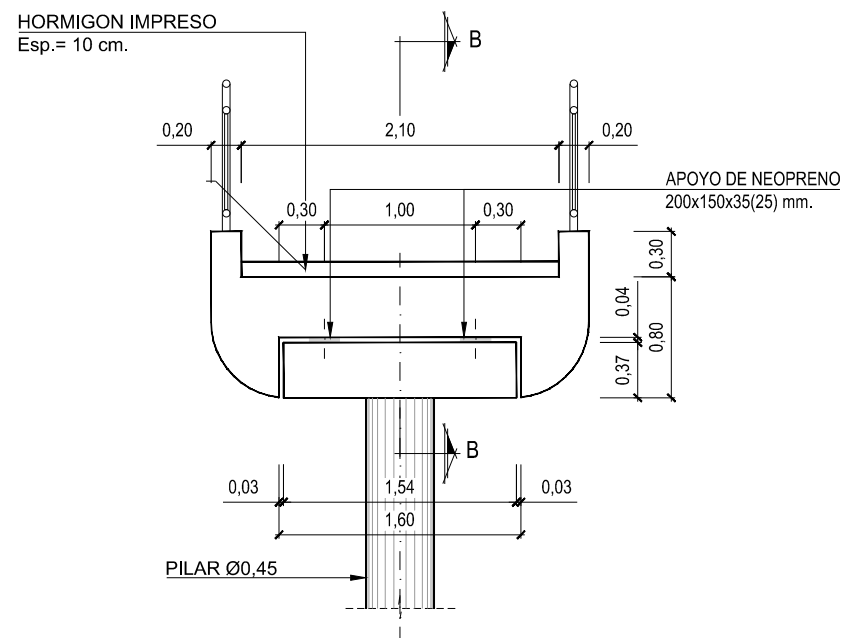
SECCIÓN TIPO: PASARELA (POR EJE DE APOYOS) ESCALA: 1/50
