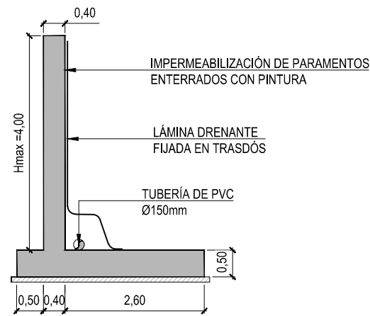
MURO TIPO 1 ESCALA: 1/100
