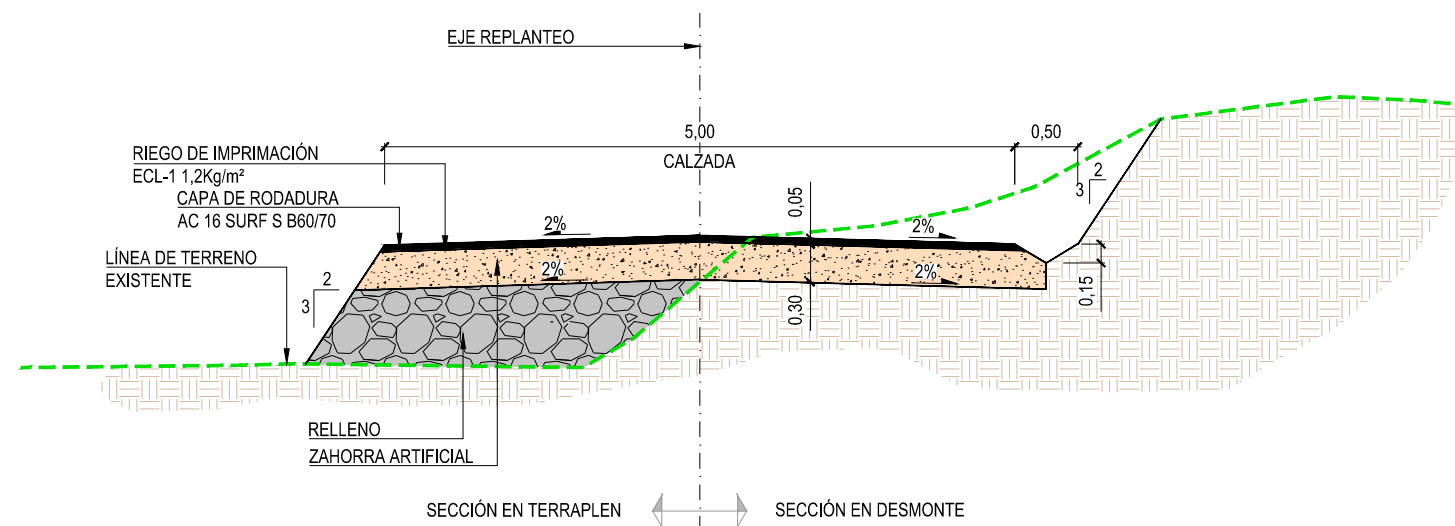
SECCIÓN TIPO: VIAL (ANCHO = 5m) ESCALA: 1/60
