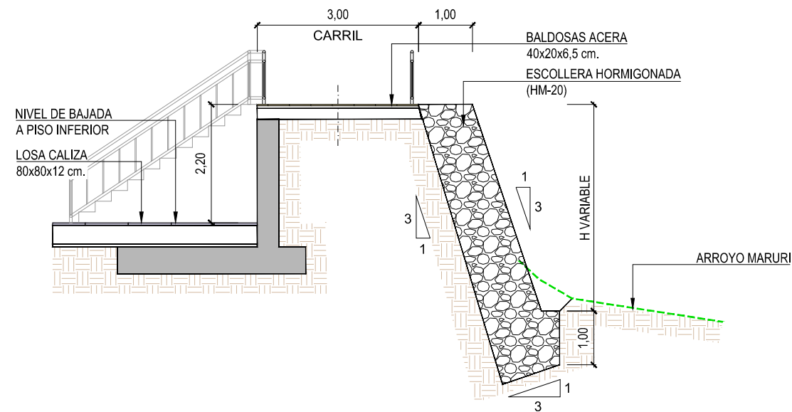
SECCIÓN A-A: MURO DE ESCOLLERA ESCALA: 1/100
