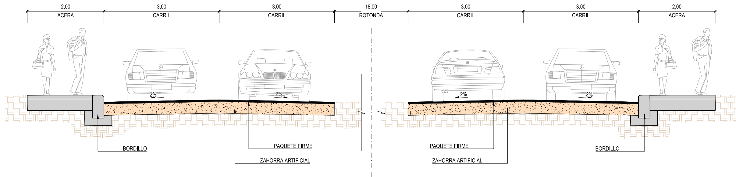
SECCIÓN TIPO: GLORIETA ORIBE (ATERNATIVA 1 Y 2) ESCALA: 1/60
