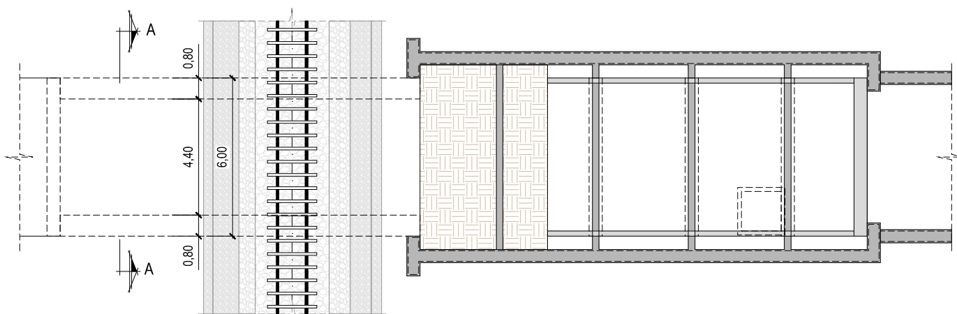
PASO INFERIOR TIPO 1. PLANTA ESCALA: 1/200
