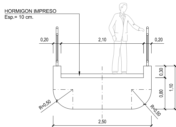
SECCIÓN TIPO: PASARELA ESCALA: 1/50
