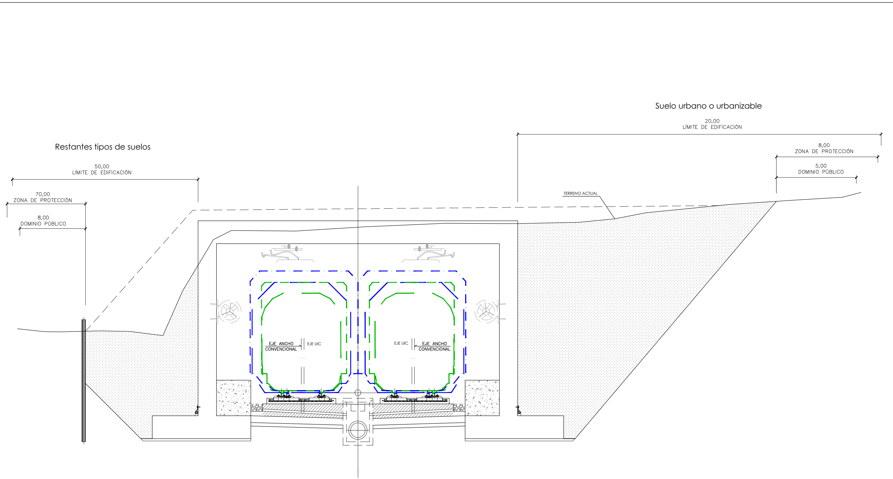
Sección tipo falso túnel
