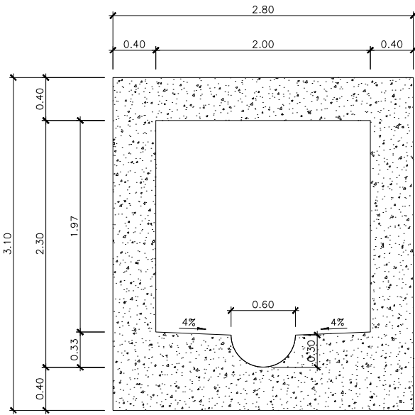
SECCIÓN TIPO COLECTOR 1 (TRAMO 1.A) 2.00x2.30x0.30m ESCALA 1:25 (NOTA: COTAS EN m)
