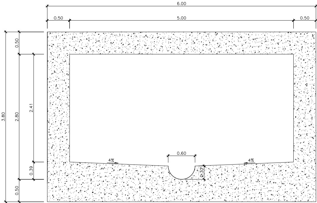
SECCIÓN TIPO COLECTOR 1 ( TRAMO 1.B) 5.00x2.80m ESCALA 1:25 (NOTA: COTAS EN m)
