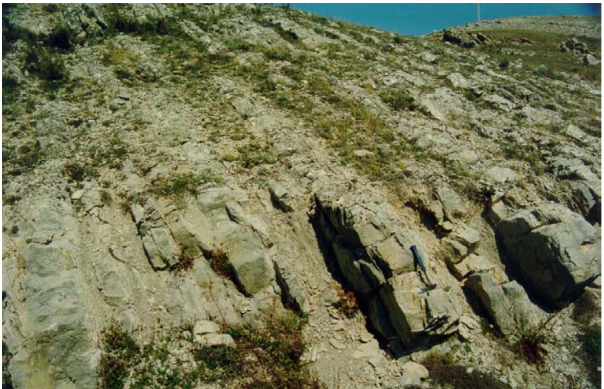
FOTO Nº 56. Alternancia rítmica de calizas, margas y margocalizas en el cerro Solera, al N de la estación de Aguilar (grupo 220).
