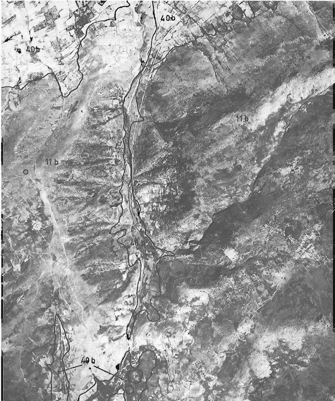
Fig. 5. Foto aérea de la parte central de la zona del puerto de Somosierra, con los grupos litológicos más importantes
