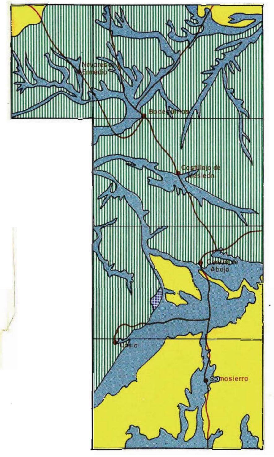
MAPA ESQUEMATICO GEOTECNICO - Escala, 1:200.000
