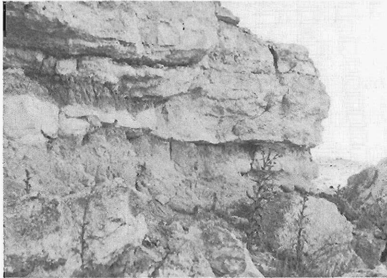
Fig. 48. Basculamiento de los bloques de caliza del páramo, por alteración de las margas de la base. Margen izquierda de la carretera a Pardilla
