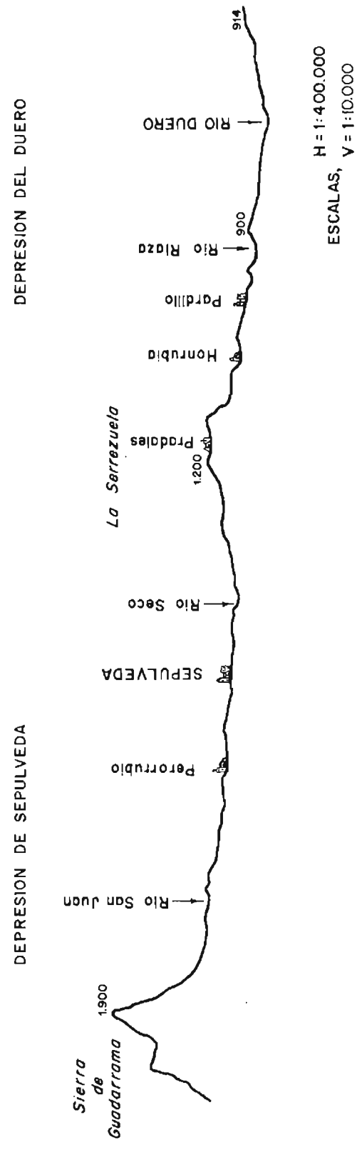
Fig. 2. Perfil topográfico del tramo
