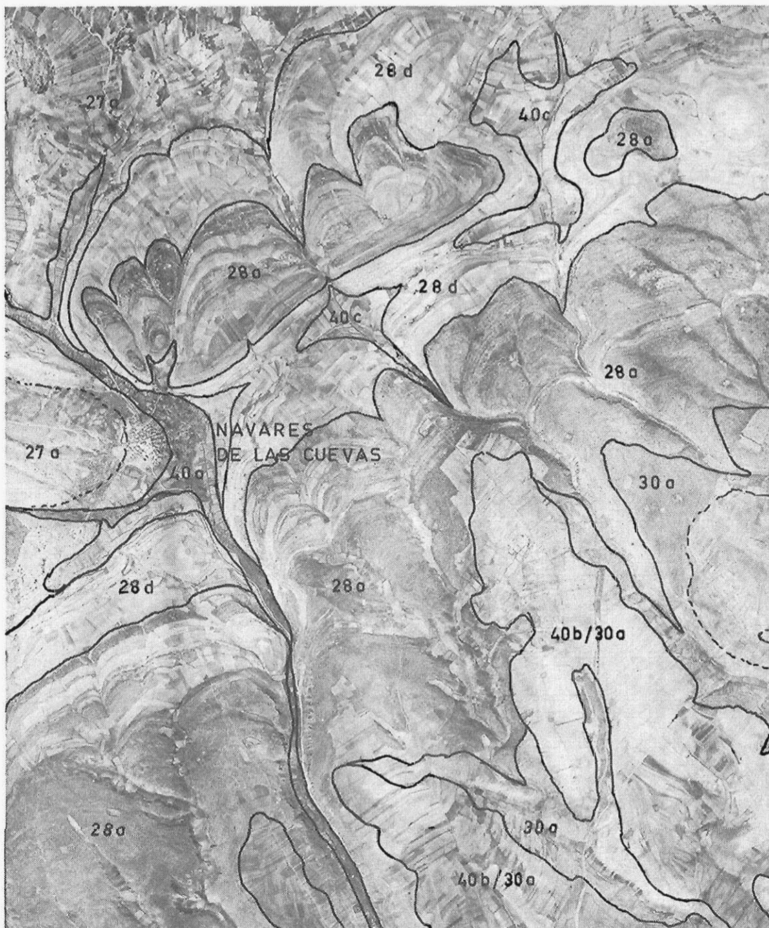
Fig. 25. Foto aérea de la parte oeste de la zona Fresno de la Fuente-N. de Honrubia de la Cuesta, con los grupos litológicos más importantes
