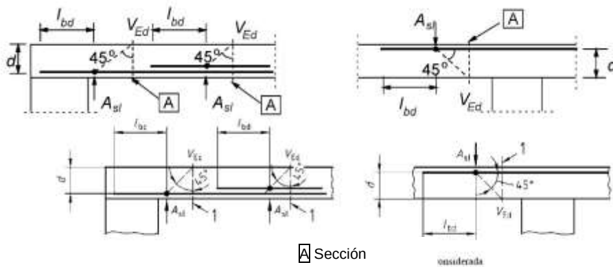
Figura A21.6.3 Definición de A_{sl} en la expresión (6.2)
