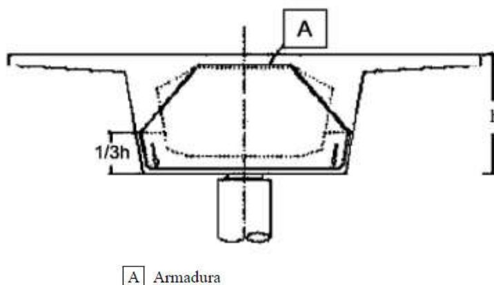
Figura A21.OO.6 Diafragmas con apoyo indirecto. Anclaje de la armadura de suspensión
