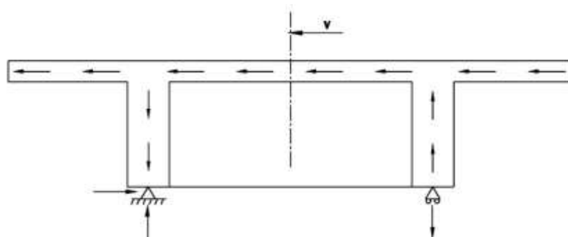
Figura A21.OO.9 Esfuerzo cortante horizontal y reacciones en los apoyos
