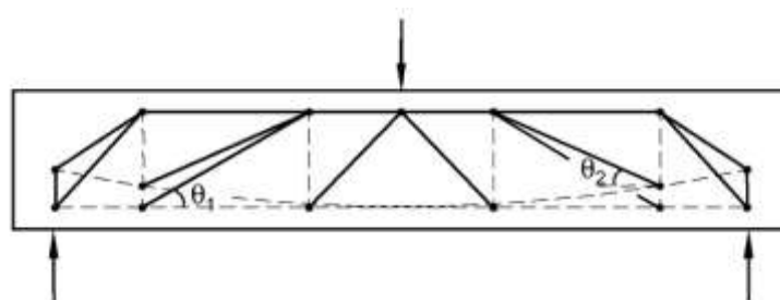
Figura A21.6.102 Superposición de modelos de resistencia a esfuerzo cortante
