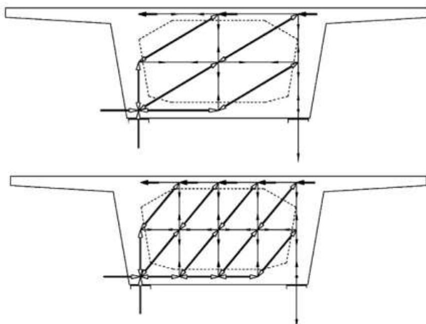
Figura A21.OO.3 Modelo de bielas y tirantes para un diafragma macizo tipo con apoyo directo sin paso de hombre
